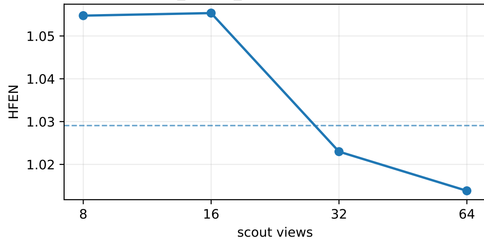
lof_flange_v3 - HFEN (k=80)
