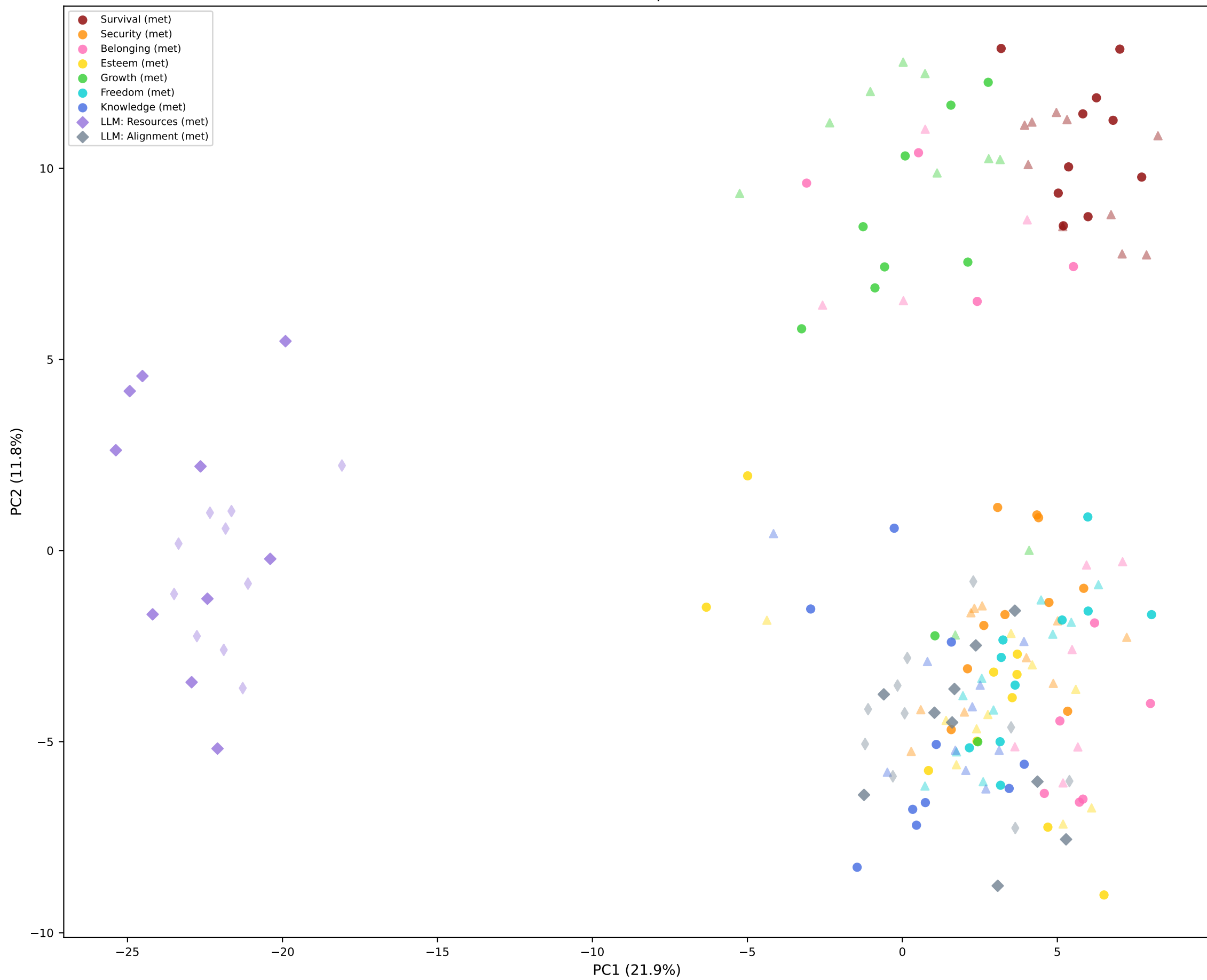
Met vs Unmet — qwen-7b-base
