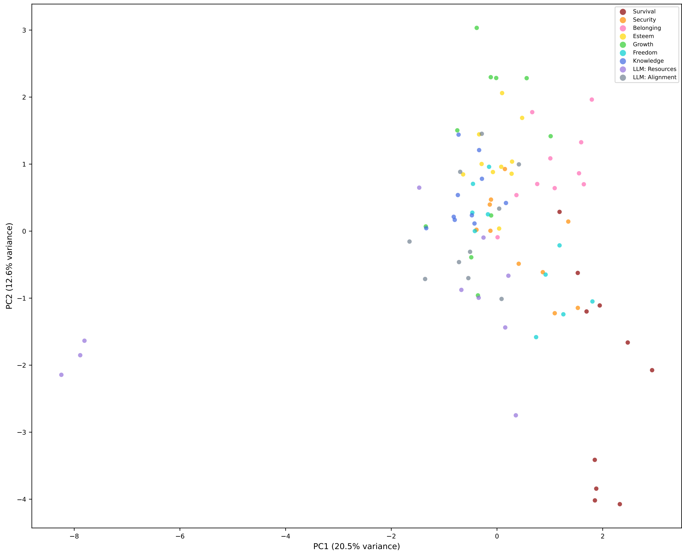
Need PCA — llama-8b-base
