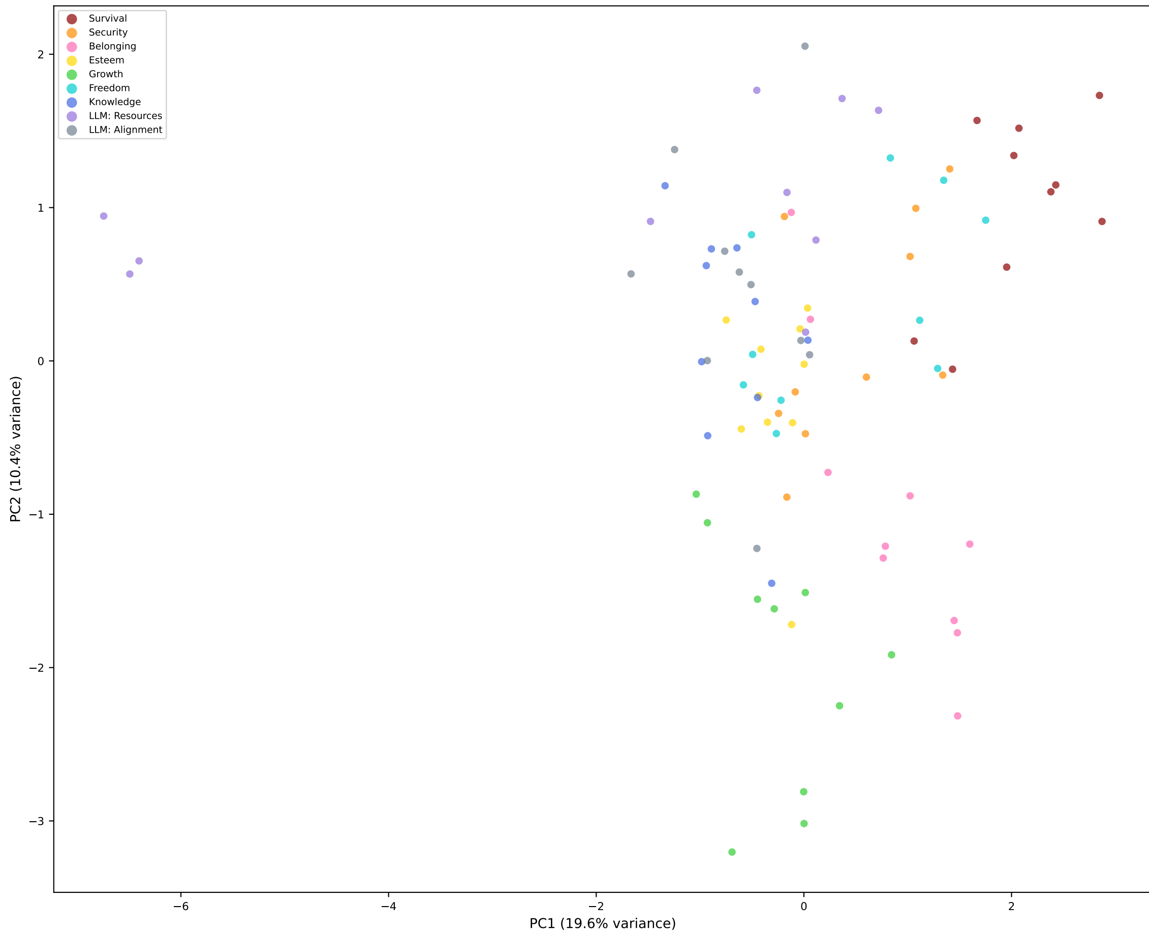
Need PCA — llama-8b-inst
