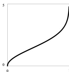
Quantils for Weibull(.,2,2)
