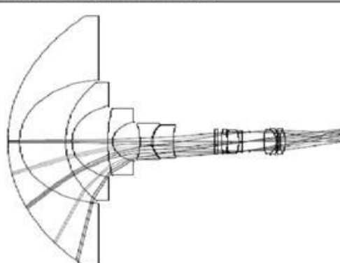
图 8: 鱼眼镜头的光学设计结构
