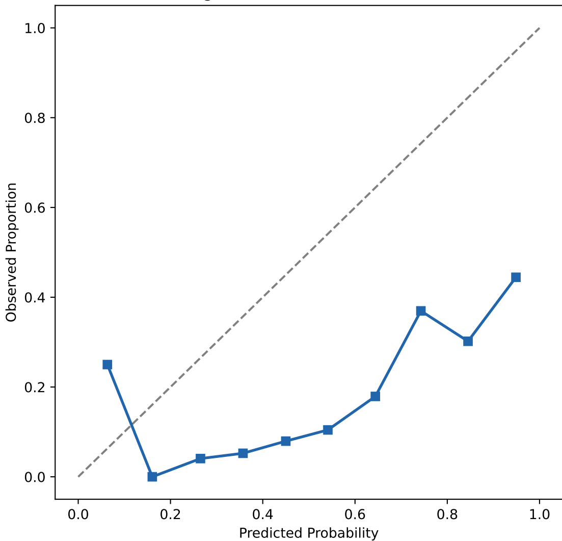
Nomogram Calibration (AUC=0.6678)
