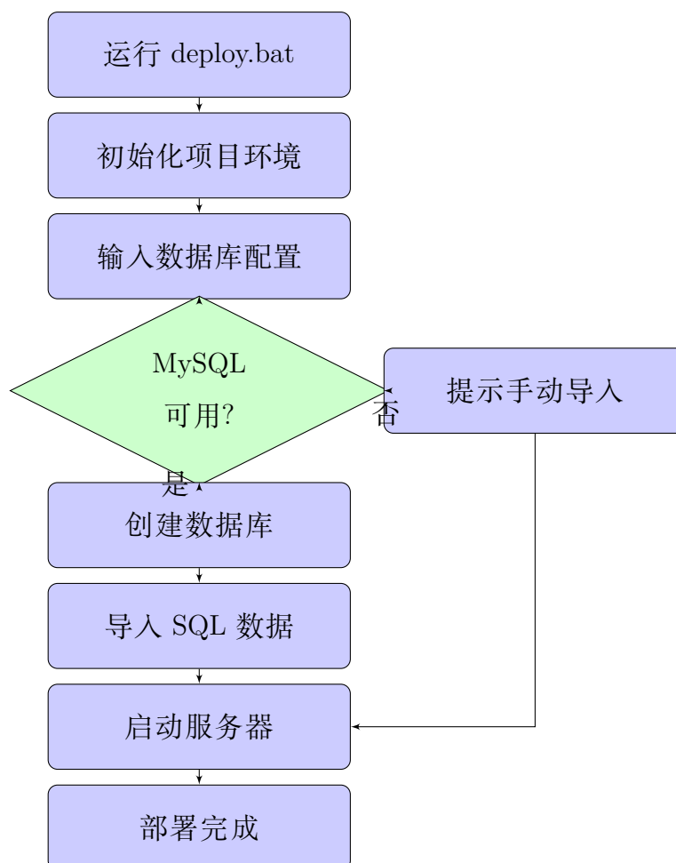
图 4: 一键部署流程图
