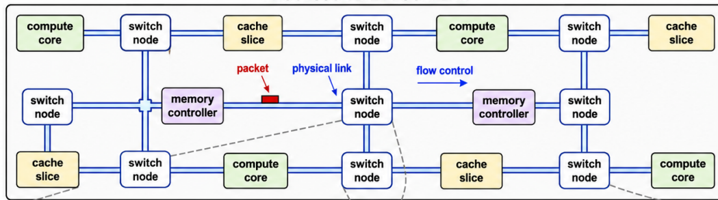
PROCESSOR DIE FLOORPLAN
