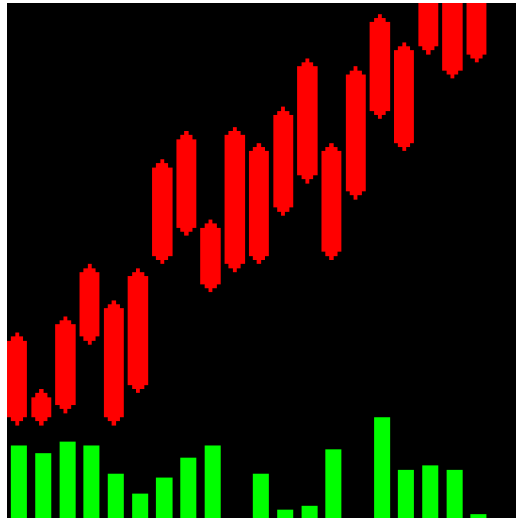
(d) Hybrid
