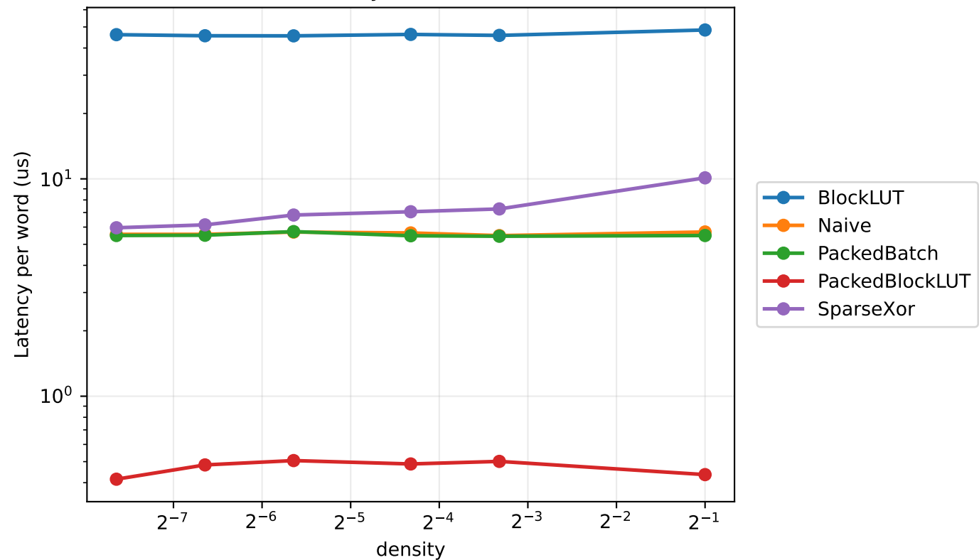
GF(2) density micro-benchmark
