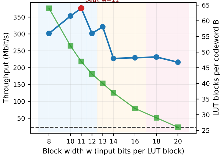
(b) BCH(511,484), r=27 , batch=10000
