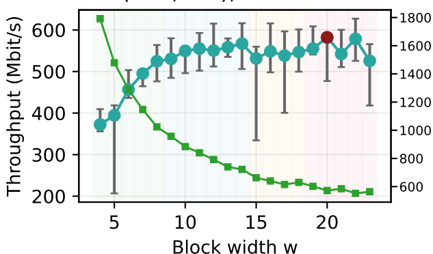
BCH(511,484), r=27: median
