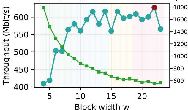
BCH(511,484), r=27: max envelope
