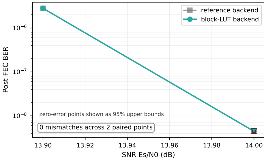
Real OFEC BER, h=16
