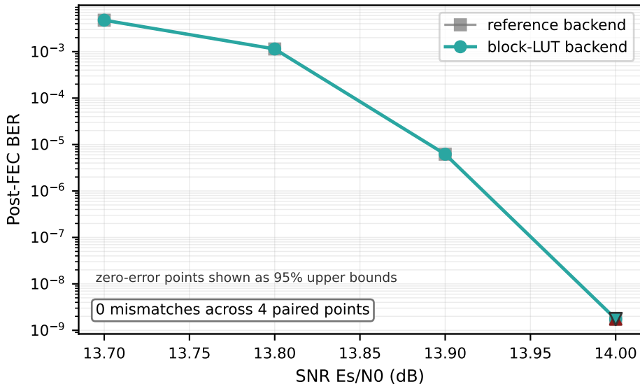
Real OFEC BER, h=10
