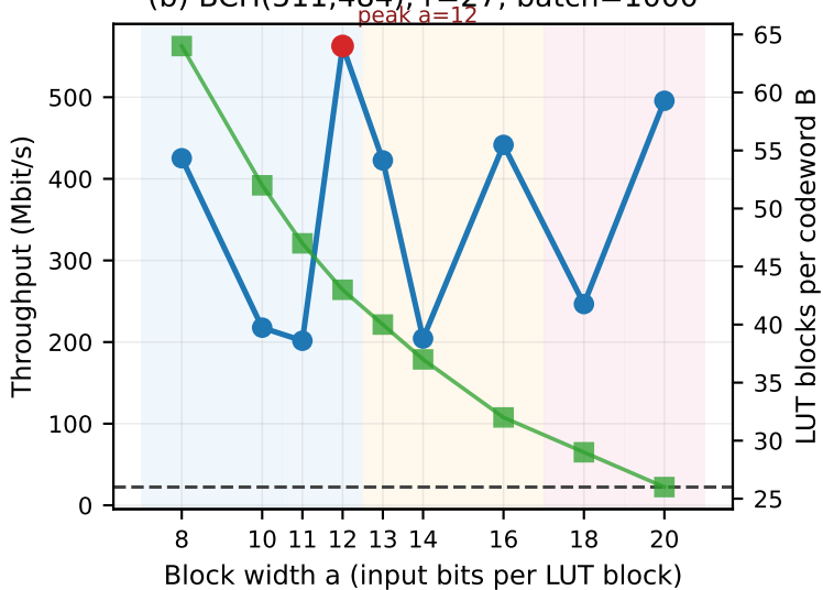
(b) BCH(511,484), r=27 , batch=1000
