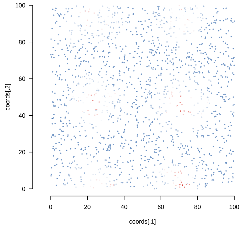
(b) local Moran (LISA)
