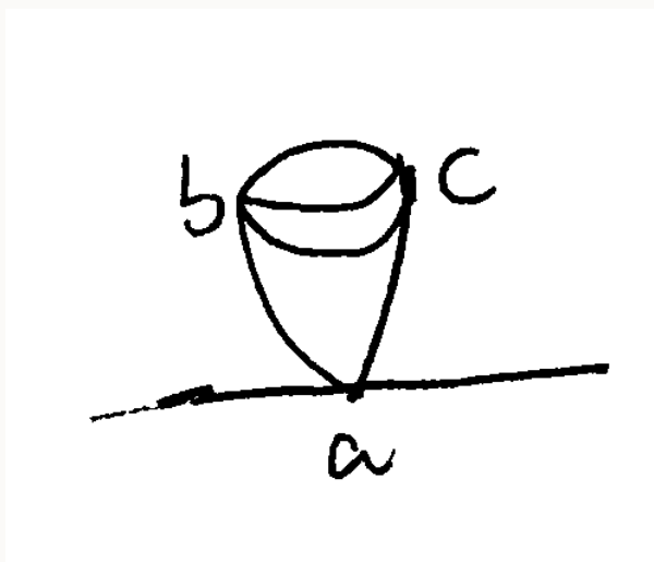
图 7.4: 存在内点置换对称性的 Feynman 图
