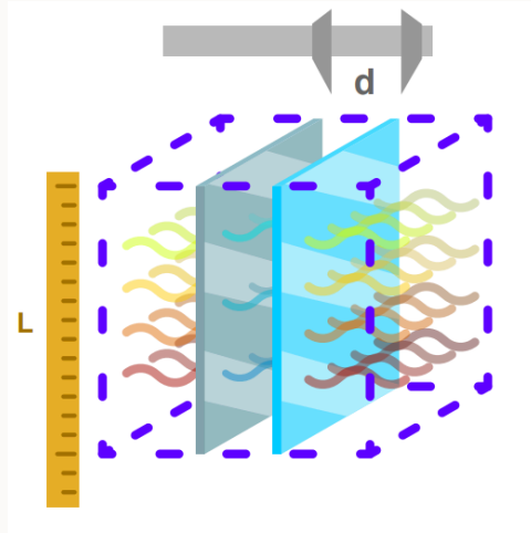
图 16.1: Casmir 效应示意图
