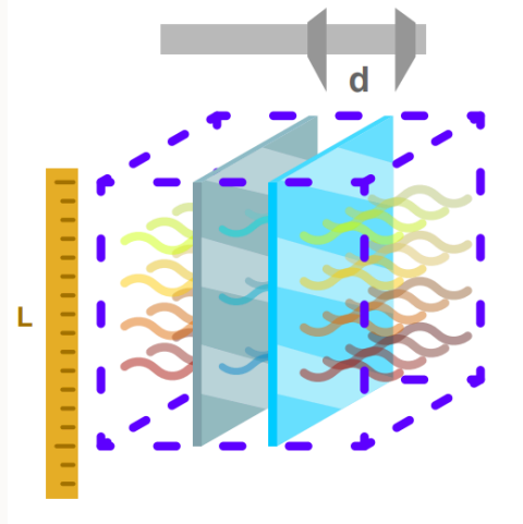
图 17.1: Casimir 效应示意图
