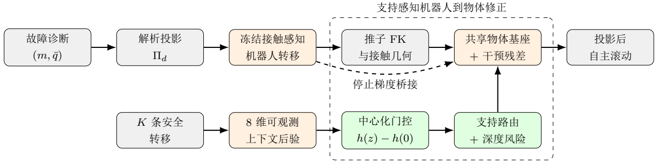
图 1: IPWM 部署图。已知损伤由解析投影强制满足；上下文门控的几何与潜变量残差只在训练干预支持之外启用，K0 精确恢复基座。
