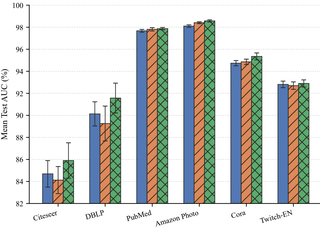
(a) Test AUC
