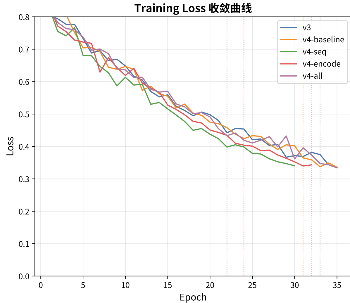
Figure 2 模型训练过程对比
