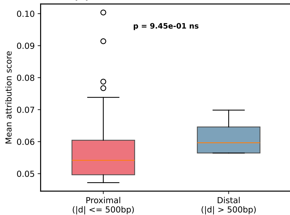
(d) Proximal vs Distal Attribution
