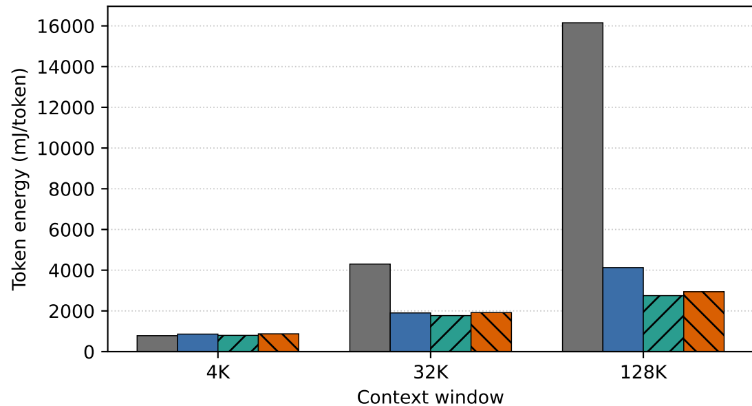
Llama2-70B
