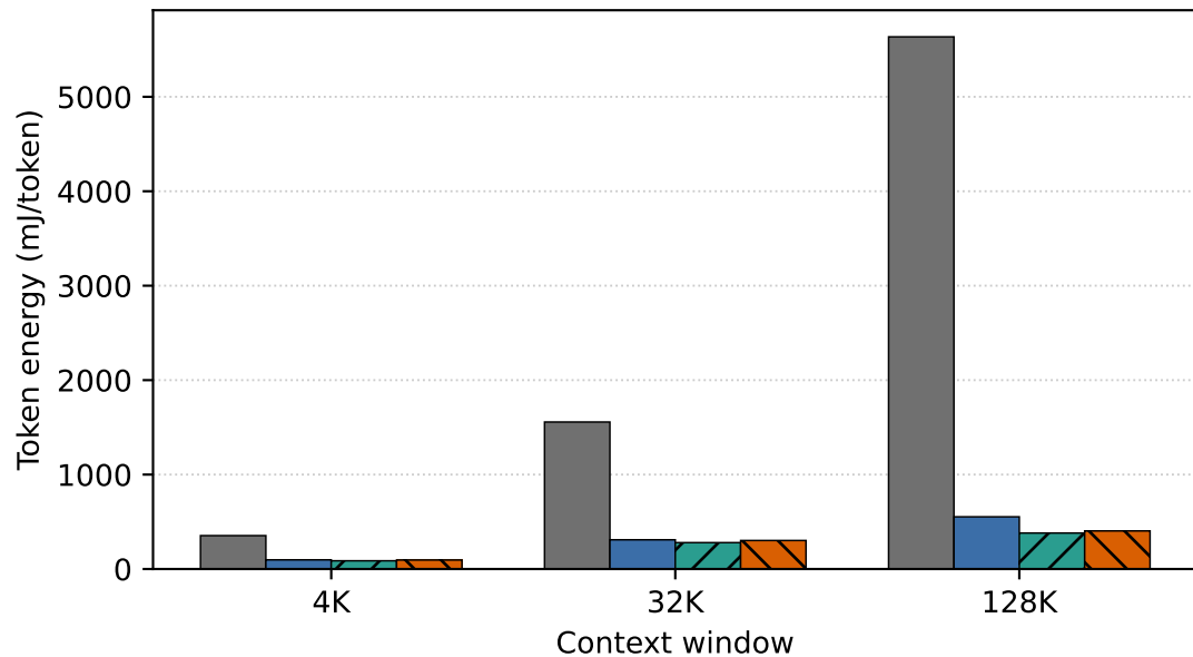
Llama2-7B
