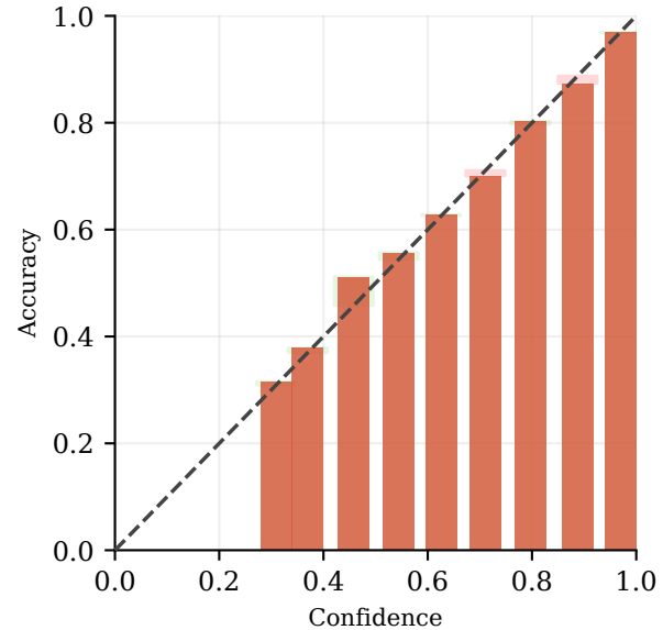
Dir.-Soft ECE = 0.2%
