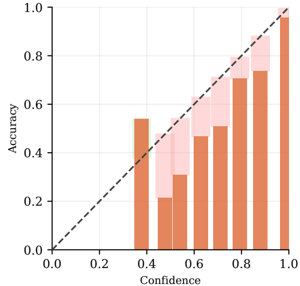
TS ECE = 4.2%
