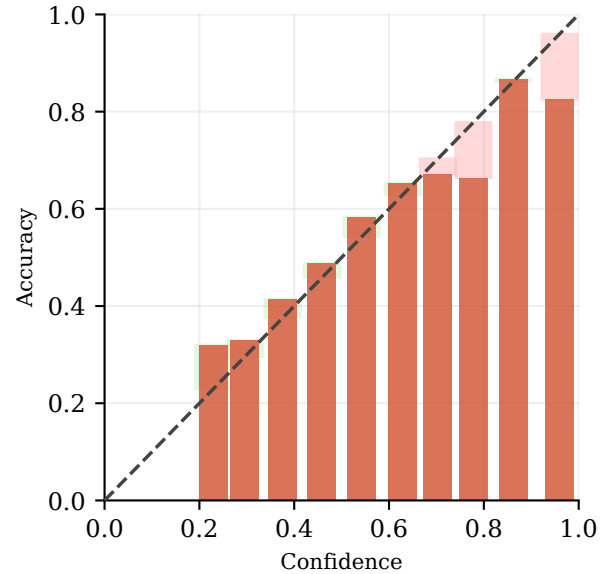
Dir.-Soft ECE = 3.8%
