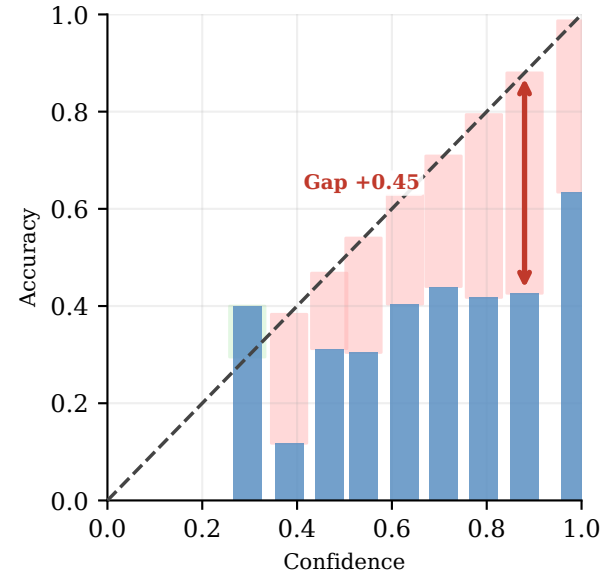
Uncal ECE = 34.3%
