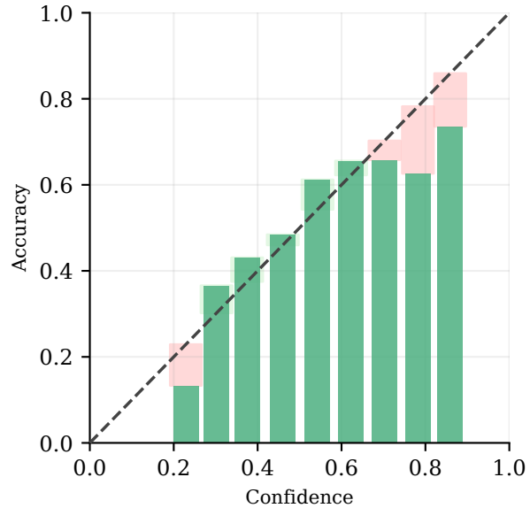
SLTS ECE = 5.3%
