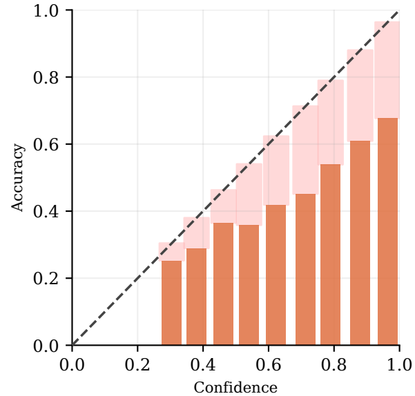
TS ECE = 24.8%
