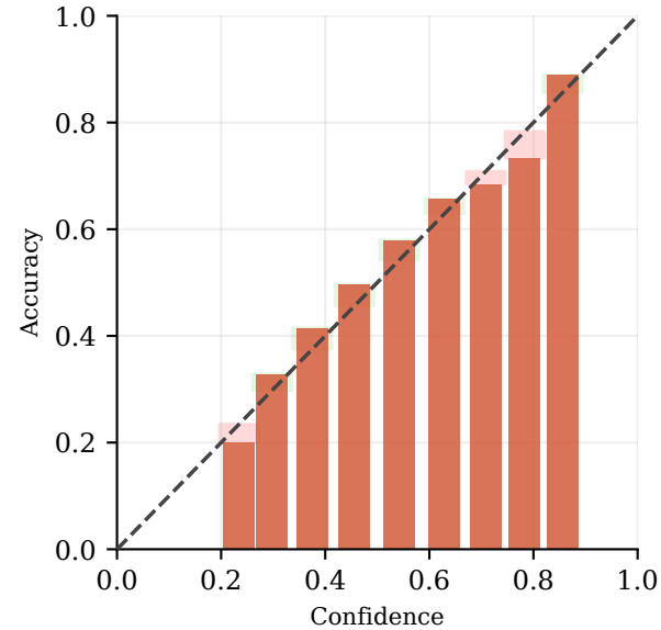
Dir.-Soft ECE = 3.1%
