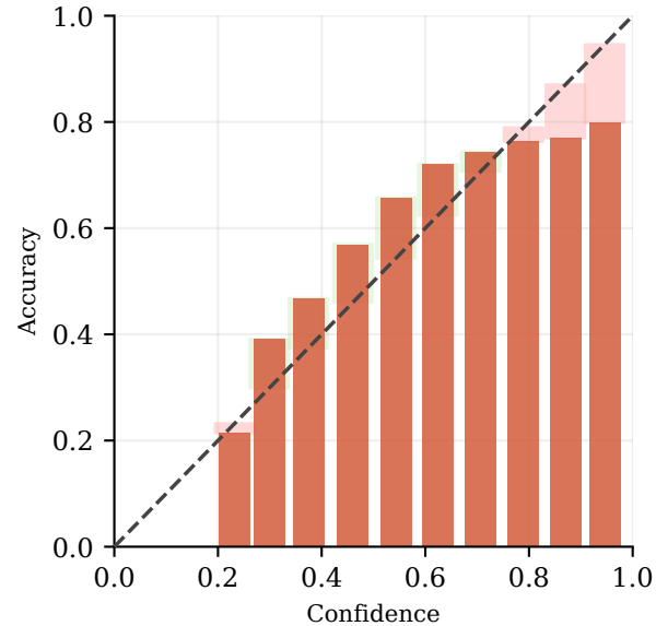
Dir.-Soft ECE = 8.2%
