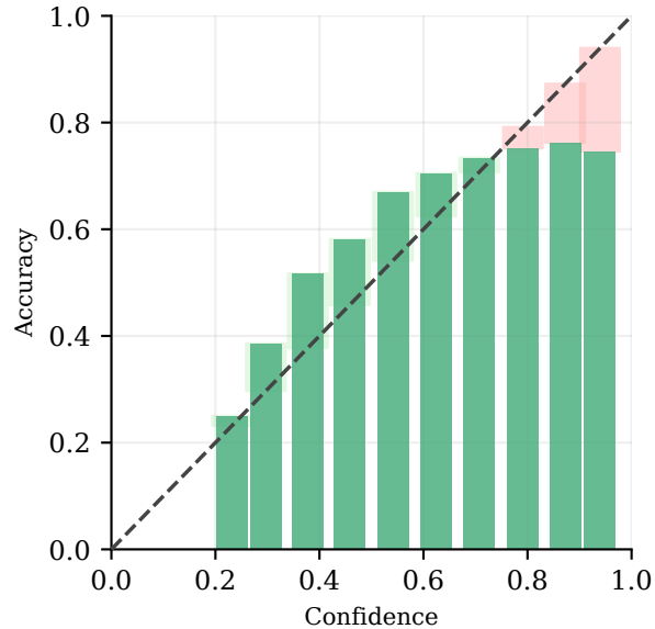
SLTS ECE = 9.4%
