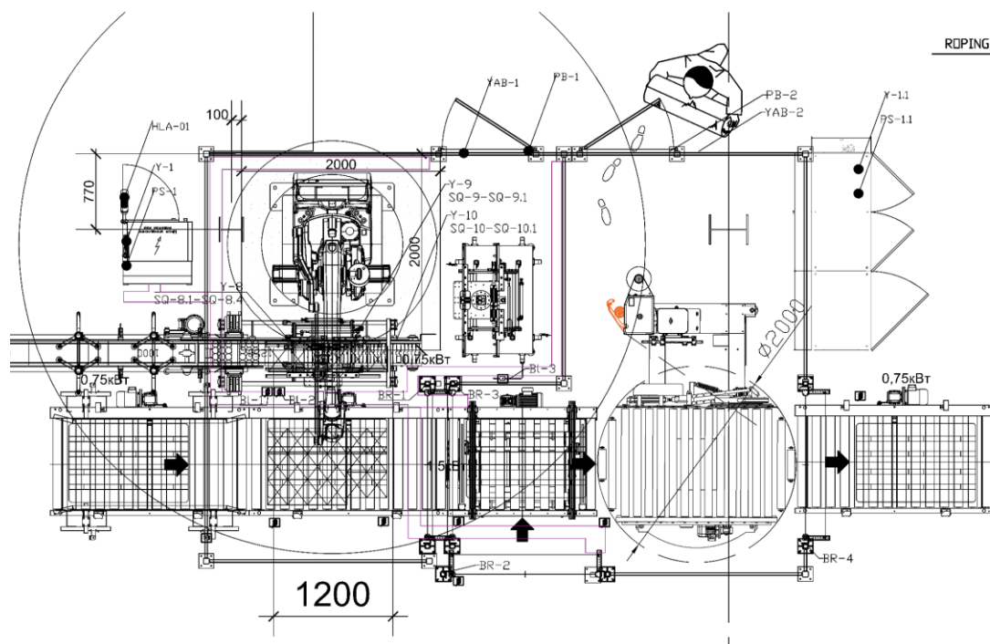
Рисунок 12 - Схема роботизированной ячейки паллетизации, использованная как исходная планировка цифровой модели
