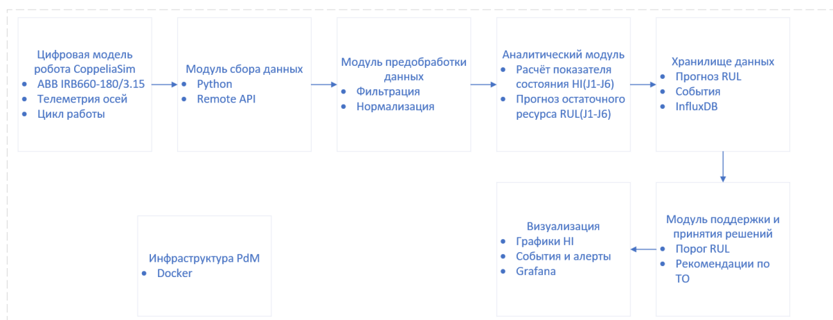
Рисунок 7 - архитектура ПАК
