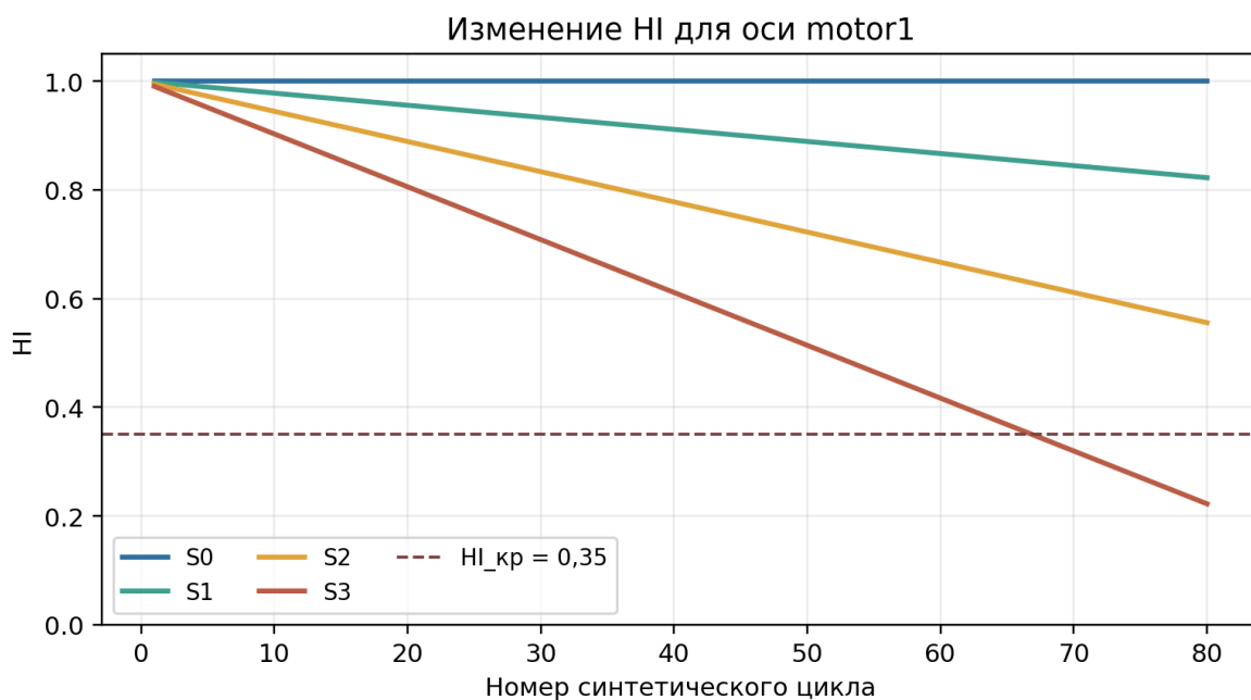
Рисунок 16 - Изменение индекса HI для motor1 по сценариям деградации
