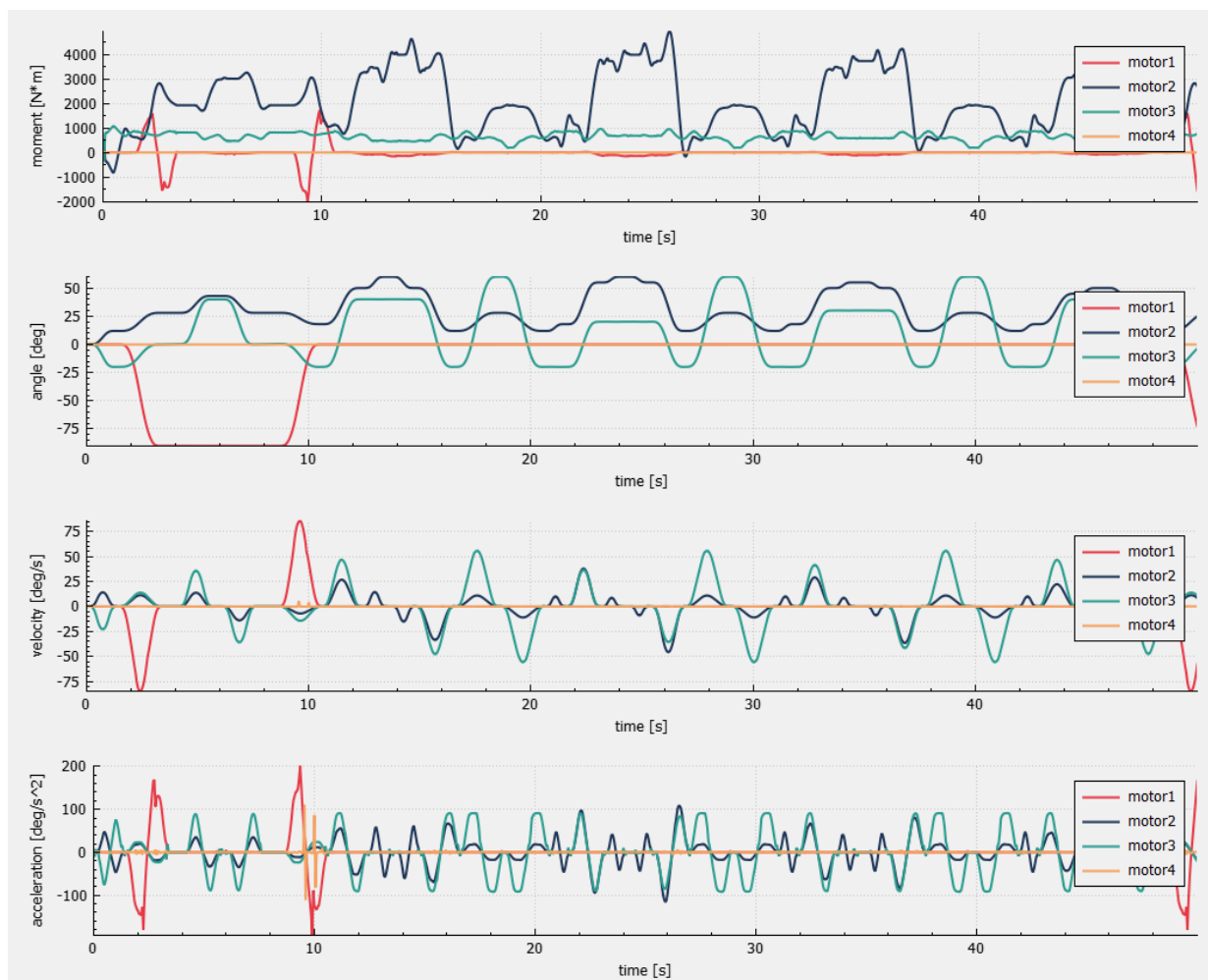
Рисунок 3 - графики телеметрии в среде CoppeliaSim
