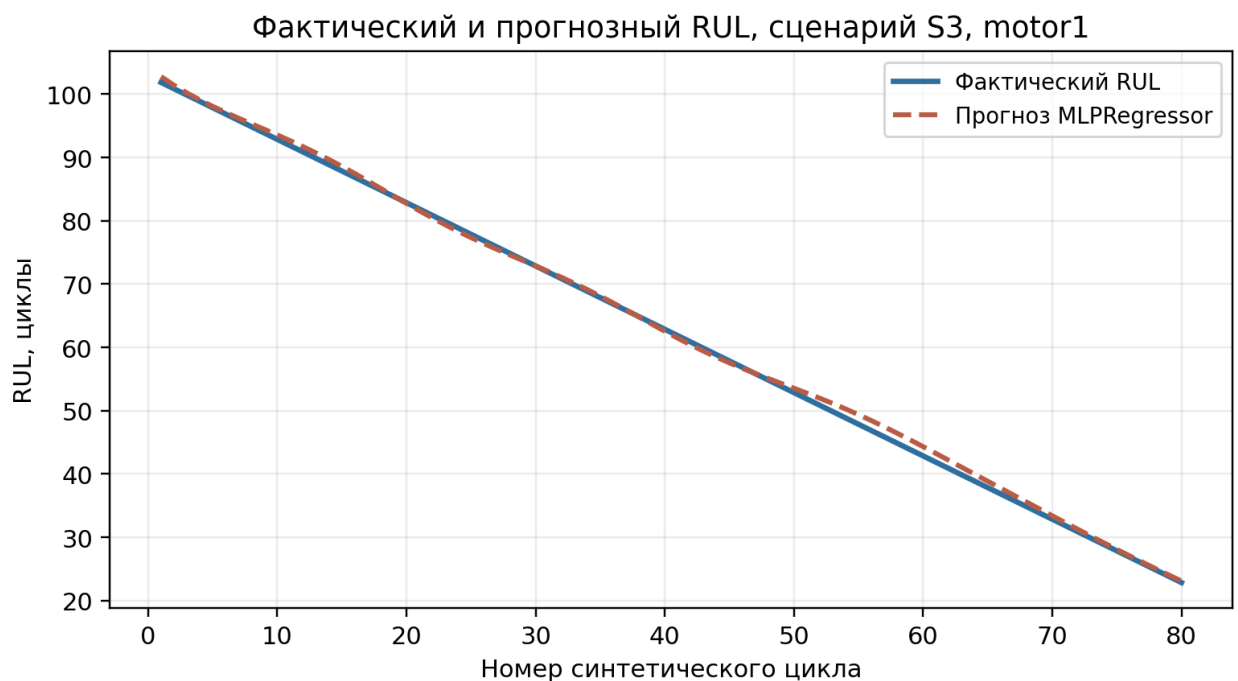
Рисунок 13 - Контрольный пример сравнения фактического и прогнозного RUL
