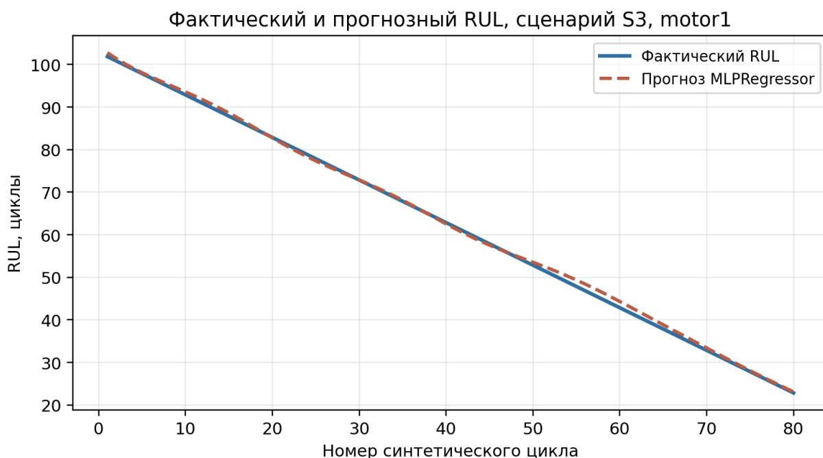
Рисунок 15 - Сравнение фактического и прогнозного RUL для сценария S3, motor1
