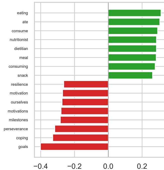
iter 3→4
