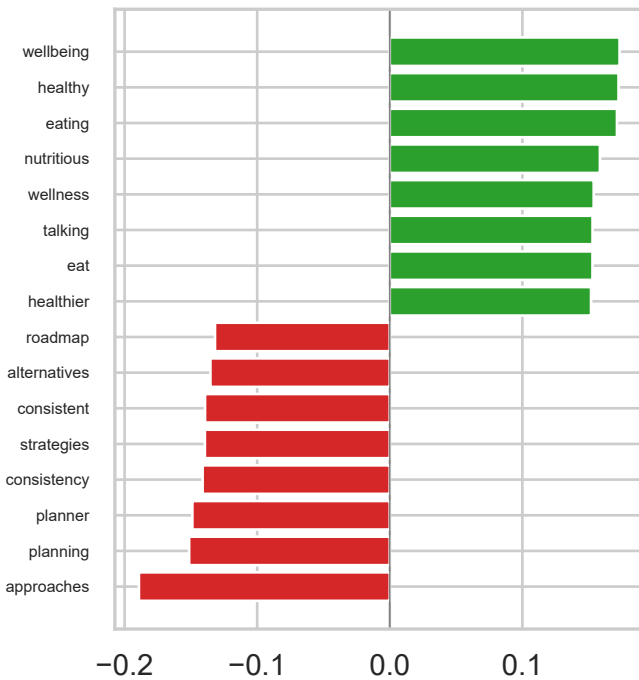
iter 1→2
