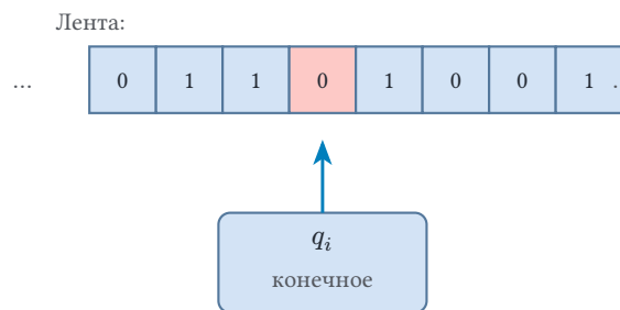
Рис. 108. Схема машины Тьюринга.
