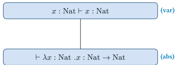
Рис. 115. Дерево вывода типа для тождественной функции.
