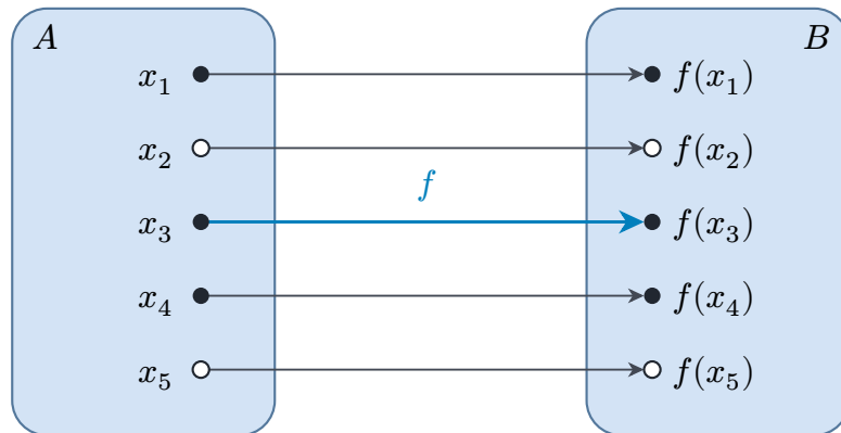
Рис. 110. Сведение A \leq_m B через функцию f .
