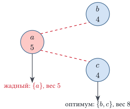
Рис. 84. Контрпример к жадному алгоритму.
