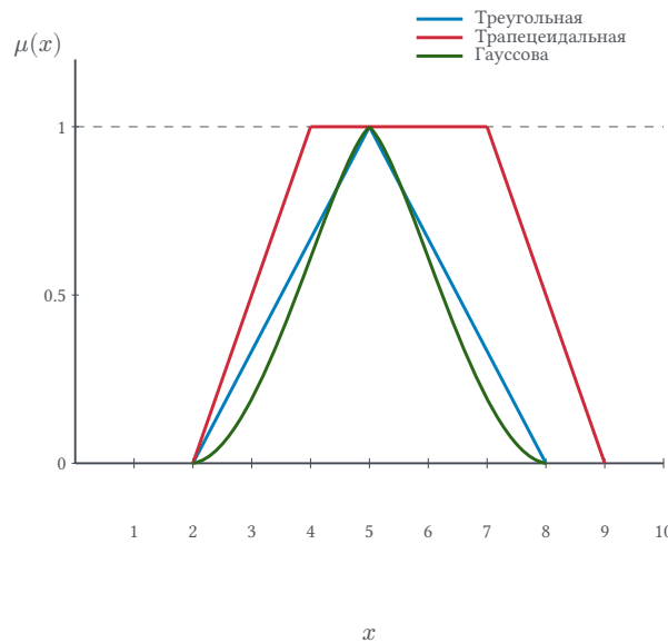
Рис. 134. Функции принадлежности: треугольная (2, 5, 8), трапецидальная (2, 4, 7, 9) и гауссова с центром 5.
