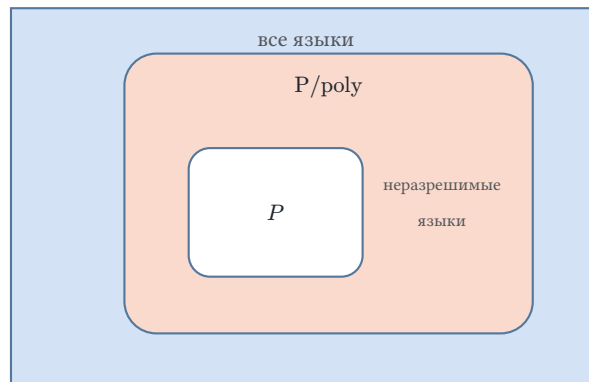
Рис. 64. Вложенность классов P \subseteq P/poly .
