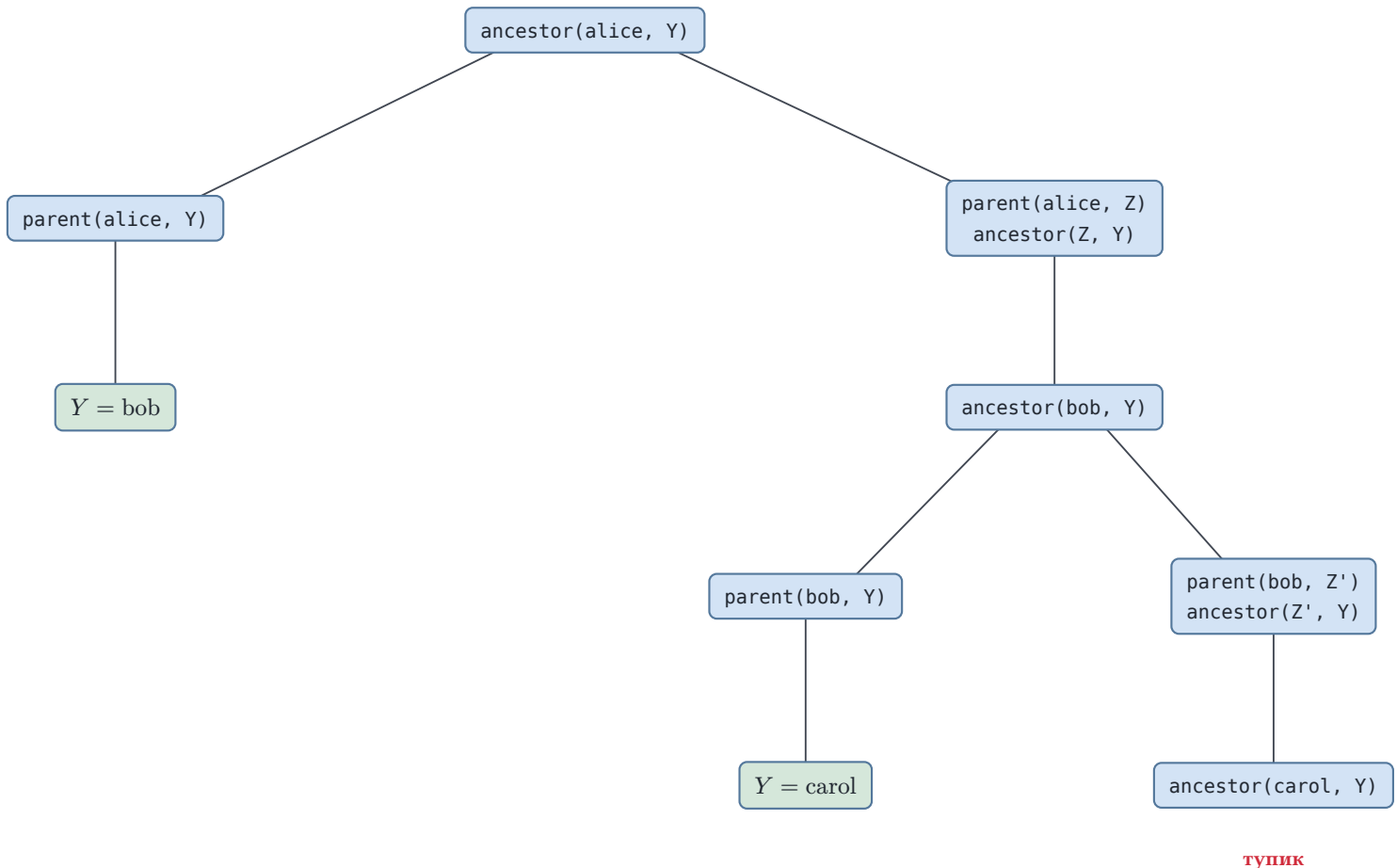
Рис. 82. SLD-дерево запроса ?- ancestor(alice, Y).
