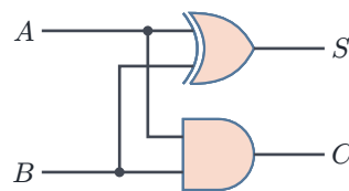
Рис. 59. Полусумматор.
