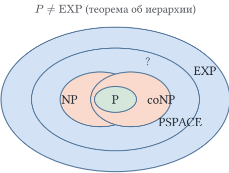
Рис. 120. Основные классы сложности.
