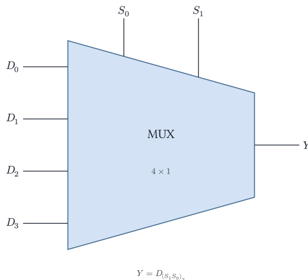
Рис. 61. Мультиплексор 4 \times 1 .
