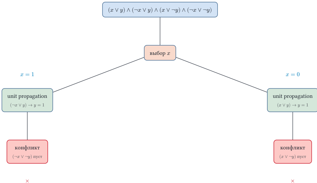
Рис. 76. DPLL-дерево поиска с возвратом.
