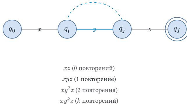
Рис. 105. Идея леммы о накачке: повторяющееся состояние образует цикл.
