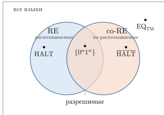
Рис. 112. Карта RE и co-RE: разрешимые — в линзе, EQ_{TM} — снаружи обоих классов.
