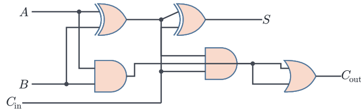
Рис. 60. Полный сумматор.
