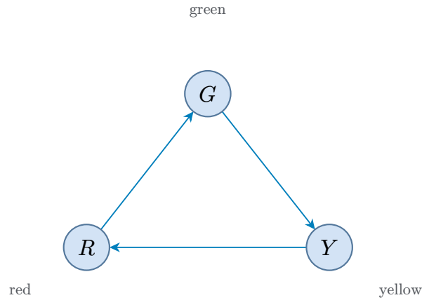
Рис. 130. Модель Крипке: цикл переходов светофора.
