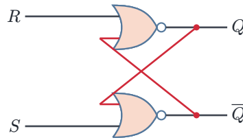
Рис. 62. SR-защёлка из двух перекрёстно соединённых вентилях NOR.
