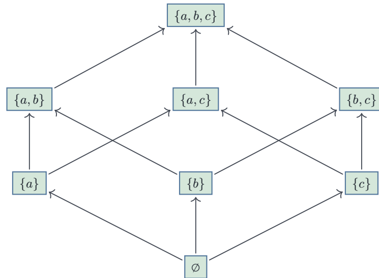
Рис. 23. Диаграмма Хассе для \mathcal{P}(\{a, b, c\}) , упорядоченного по включению.
