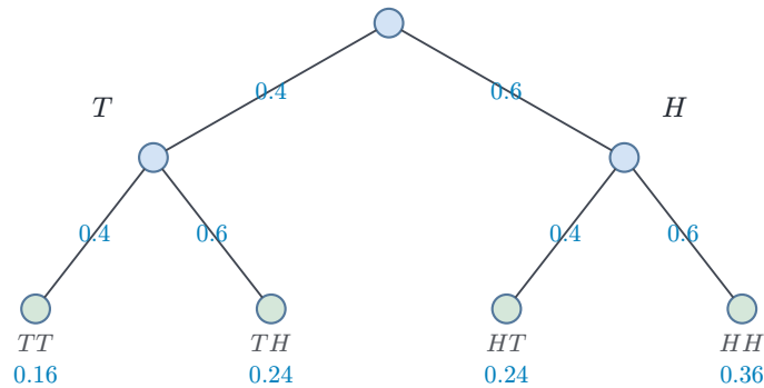
Рис. 94. Дерево вероятностей для двукратного бросания монеты.
