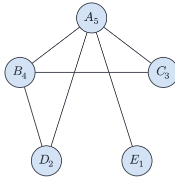
Рис. 12. Пороговый граф с весами A_5, B_4, C_3, D_2, E_1 и порогом \theta = 6 .
