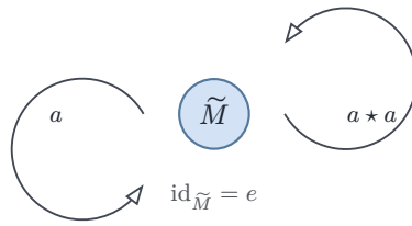
Рис. 136. Один объект, стрелки — элементы, композиция — операция.
