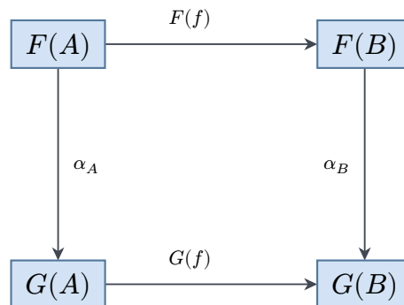
Рис. 141. Квадрат естественности: два пути из F(A) в G(B) .
