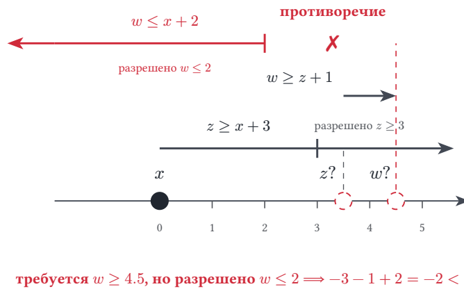
Рис. 79. Координатное прочтение примера с отрицательным циклом.
