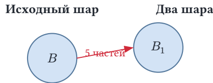
Рис. 100. Из одного шара — два того же радиуса.
