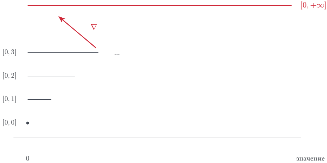
Рис. 123. Widening для цикла со счётчиком.
