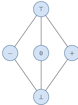
Рис. 122. Решётка домена знаков: \perp \preceq \{-, 0, +\} \preceq T .
