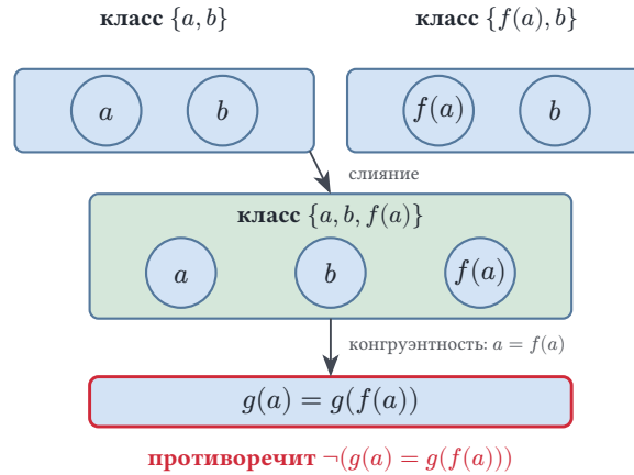
Рис. 80. Слияние классов в congruence closure.
