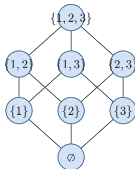
Рис. 28. Булева решётка B_3 .
