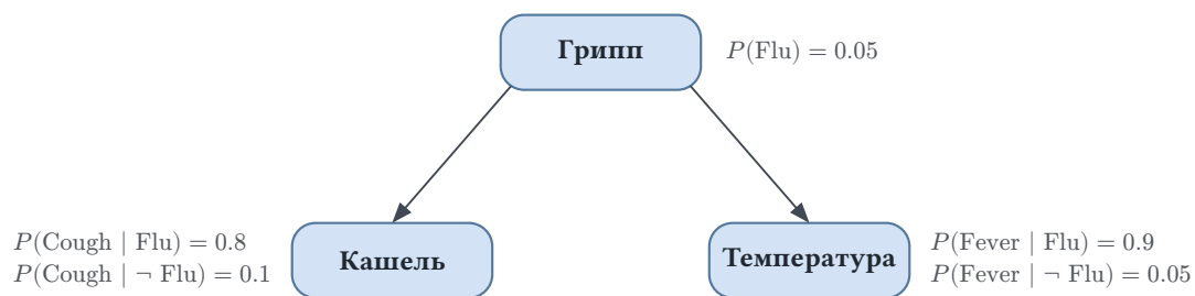
Рис. 95. Байесовская сеть: грипп влияет на кашель и температуру.
