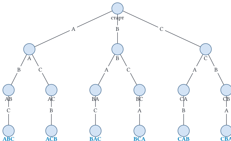
Рис. 86. Дерево решений для перестановок множества \{A, B, C\} .
