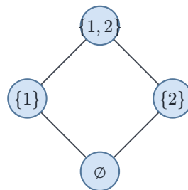
Рис. 27. Булева решётка B_2 .
