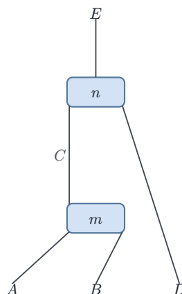
Рис. 146. Стринг-диаграмма: узлы — операции, провода — объекты, композиция идёт снизу вверх.
