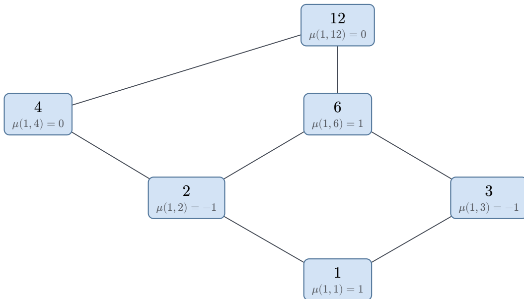
Рис. 92. Решётка делителей D_{12} со значениями \mu_{D_{12}}(1, d) .
