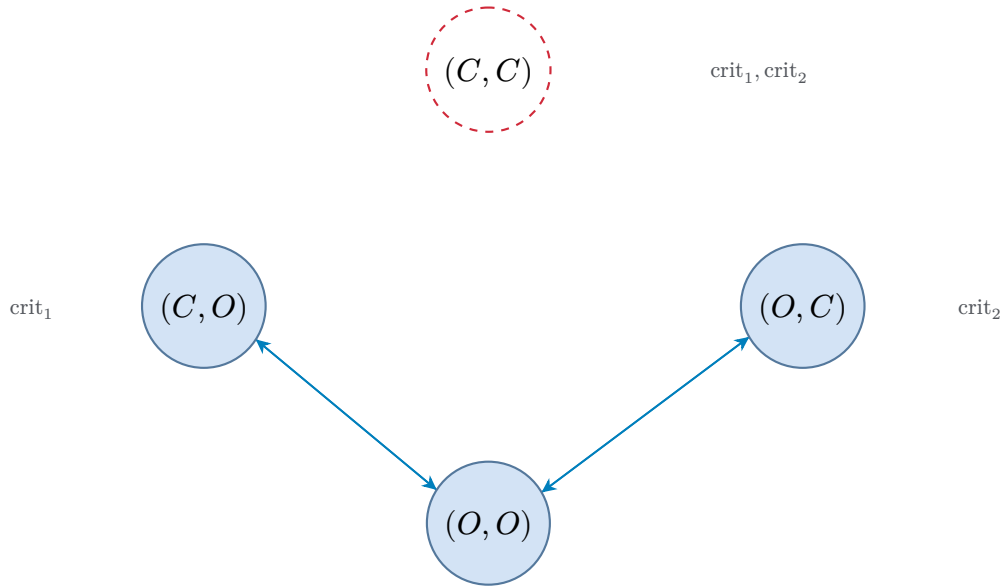
Рис. 131. Модель взаимного исключения: четыре состояния.
