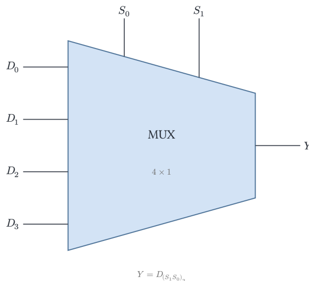
Рис. 60. Мультиплексор 4 \times 1 .
