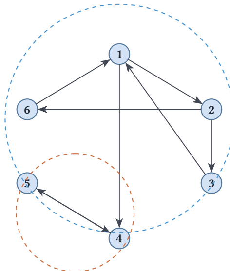
Рис. 32. Ориентированный граф.
