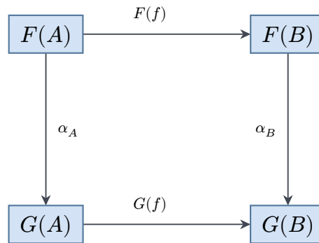
Рис. 135. Квадрат естественности: два пути из F(A) в G(B) по сторонам квадрата дают одно и то же.
