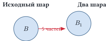
Рис. 97. Из одного шара — два того же радиуса.
