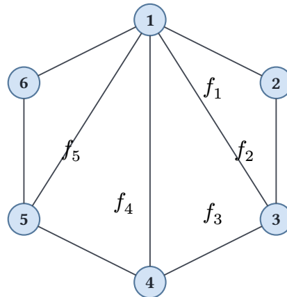
Рис. 53. Планарный граф.
