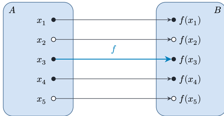
Рис. 107. Сведение A \leq_m B через функцию f .
