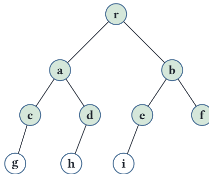
Рис. 35. Дерево.
