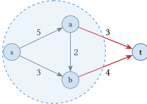
Рис. 47. Разрез A = \{s, a, b\} , B = \{t\} .
