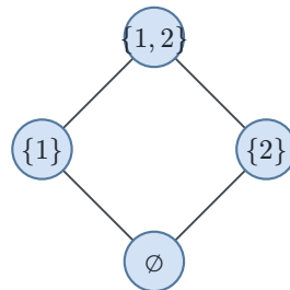
Рис. 26. Булева решётка B_2 .
