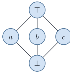
Рис. 28. Решётка M_3 (ромб).
