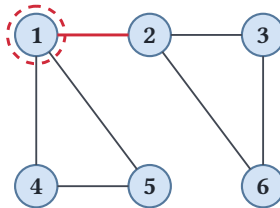
Рис. 31. Мост и точка сочленения.
