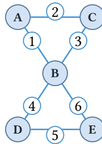
Рис. 40. Эйлеров граф-восьмёрка.
