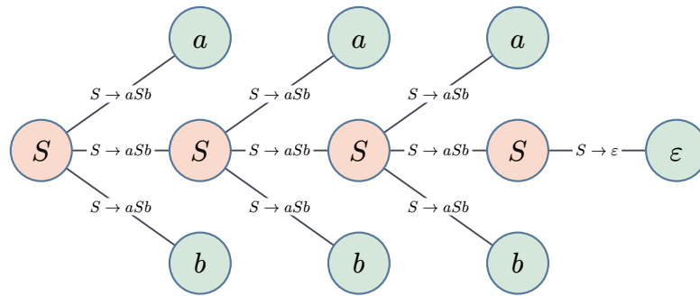
Рис. 103. Дерево разбора слова a^3b^3 .
