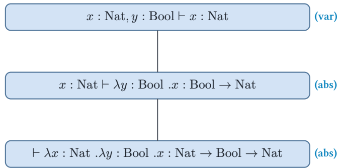
Рис. 112. Дерево вывода типа для комбинатора K .
