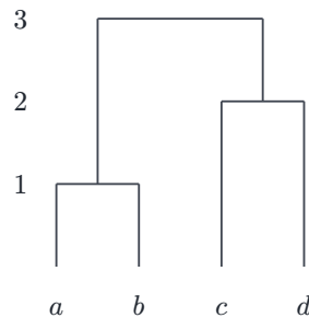
Рис. 15. Дендрограмма четырёх точек: a и b сливаются на высоте 1, c и d — на высоте 2, все вместе — на высоте 3.
