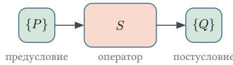
Рис. 120. Контракт: предусловие, оператор, постусловие.
