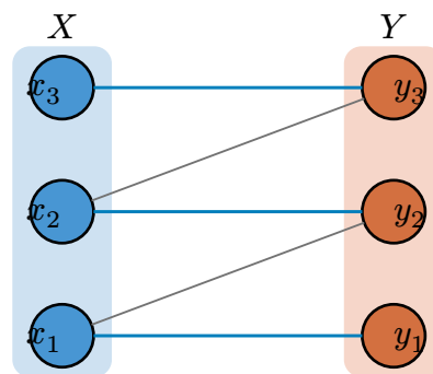
Рис. 43. Двудольный граф с максимальным паросочетанием (выделено жирным).
