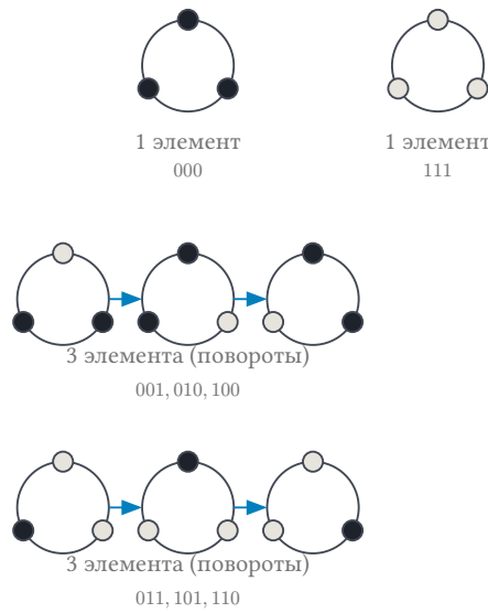
Рис. 87. Четыре орбиты ожерелий из трёх бусин двух цветов относительно циклических сдвигов.
