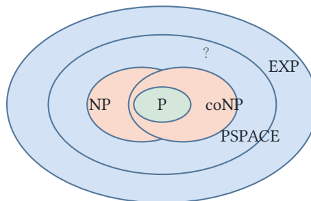
Рис. 116. Основные классы сложности.
