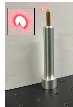
Abbildung 10: Die Justierspitze schneidet bei optimaler Justage ein Viertel des Strahlquerschnitts aus.
