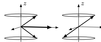
Abbildung 15: Die Addition von zwei Vektoren |s = 1/2, m_s = 1/2\rangle und |s = 1/2, m_s = -1/2\rangle kann sowohl einen Vektor |S = 1, m_S = 0\rangle ergeben (links) als auch |S = 0, m_S = 0\rangle (rechts).
