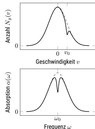
Abbildung 6: oben: Ein Laser der Frequenz \omega = \omega_0(1 - v_0/c_0) brennt ein Loch in die spontaner Maxwell-förmige Geschwindigkeitsverteilung.
