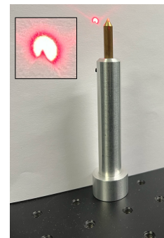
Abbildung 9: Die Justierspitze schneidet bei optimaler Justage ein Viertel des Strahlquerschnitts aus.
