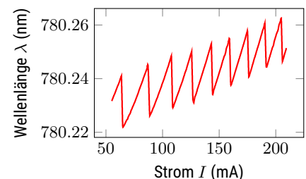
Abbildung 4: Exemplarischer Zusammenhang zwischen Laserwellenlänge und Laserstrom (aus dem Datenblatt des Herstellers).
