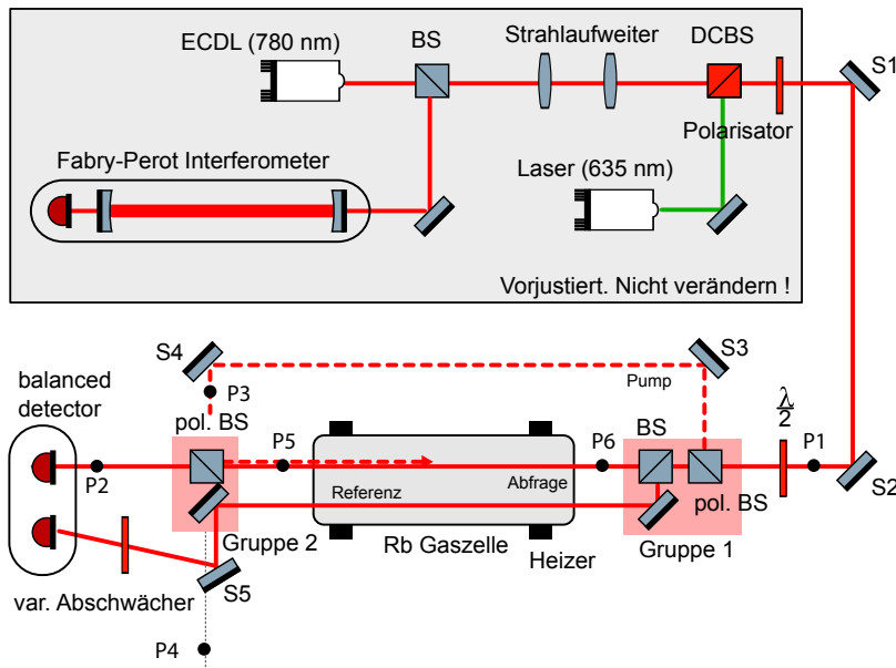
Abbildung 10: Versuchsaufbau. In den Baugruppen 1 und 2 sind die Elemente auf einer gemeinsamen Platte vorjustiert. Spiegel (S), Strahlteiler (BS), Farbteiler (DCBS), polarisierender Strahlteiler (pos. BS), Halbwellenplatte ( \lambda/2 )
