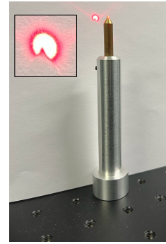
Abbildung 9: Die Justierspitze schneidet bei optimaler Justage ein Viertel des Strahlquerschnitts aus.
