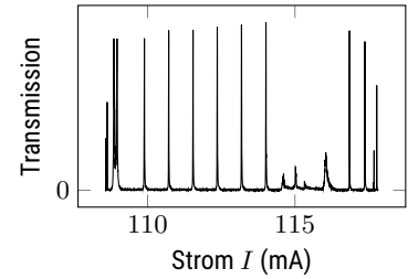
Abbildung 5: Transmission durch das Fabry-Perot-Interferometer. Bei etwa 109 mA und 115 mA sind Modensprünge zu erkennen. Der Abstand der Peaks entspricht dem FSR.
