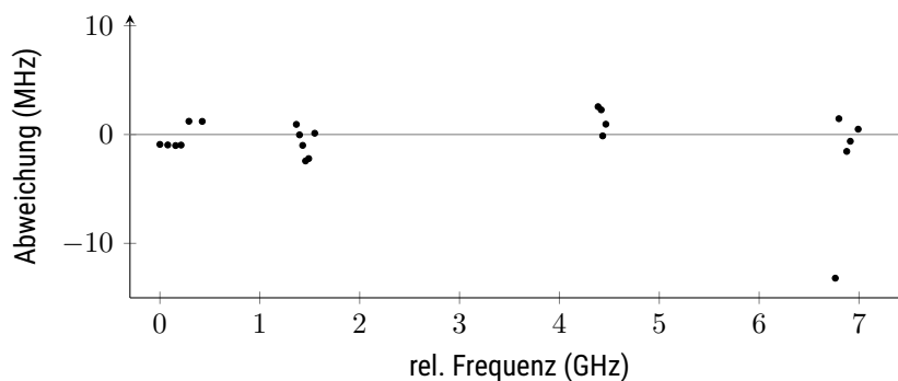
Abbildung 12: Bei optimierter Justage und Durchführung des Experiments gibt es nur eine geringe Abweichung zwischen gemessener und berechneter Linienposition.
