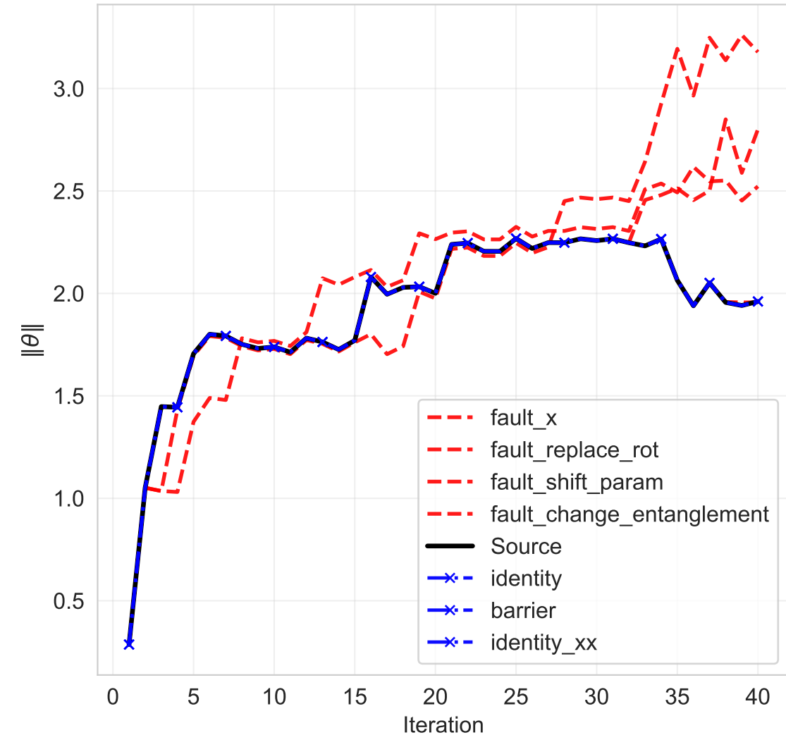
Parameter Norm Evolution
