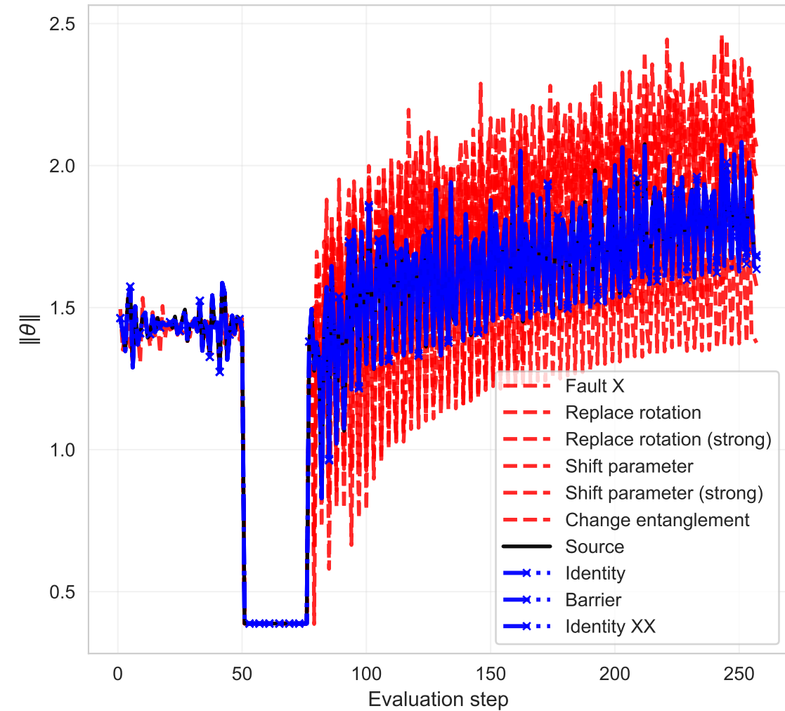
(c) Parameter Norm Evolution
