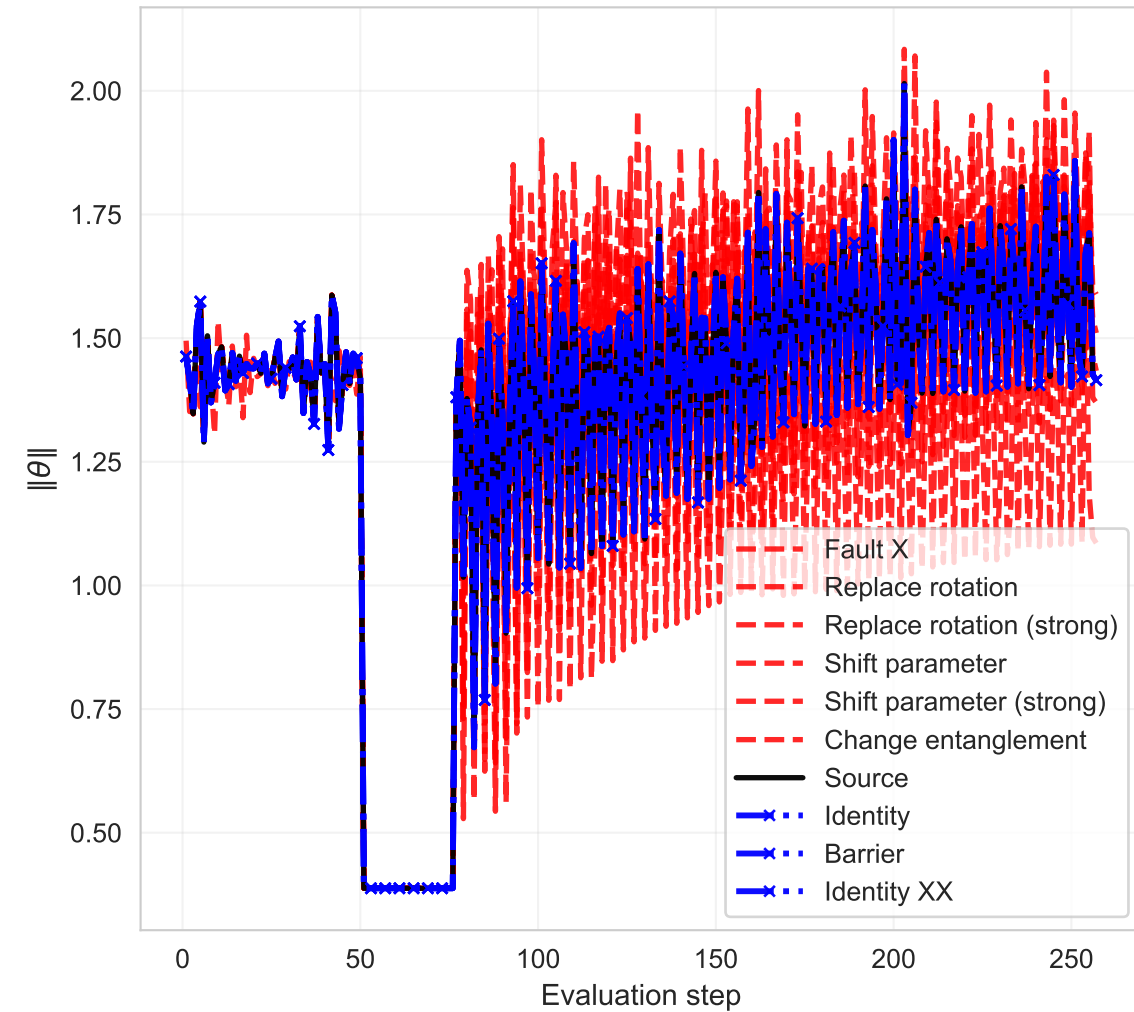
(c) Parameter Norm Evolution
