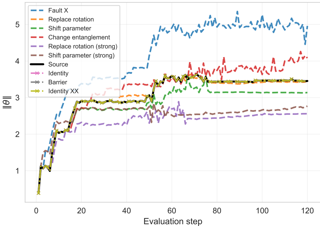
Parameter Norm Evolution
