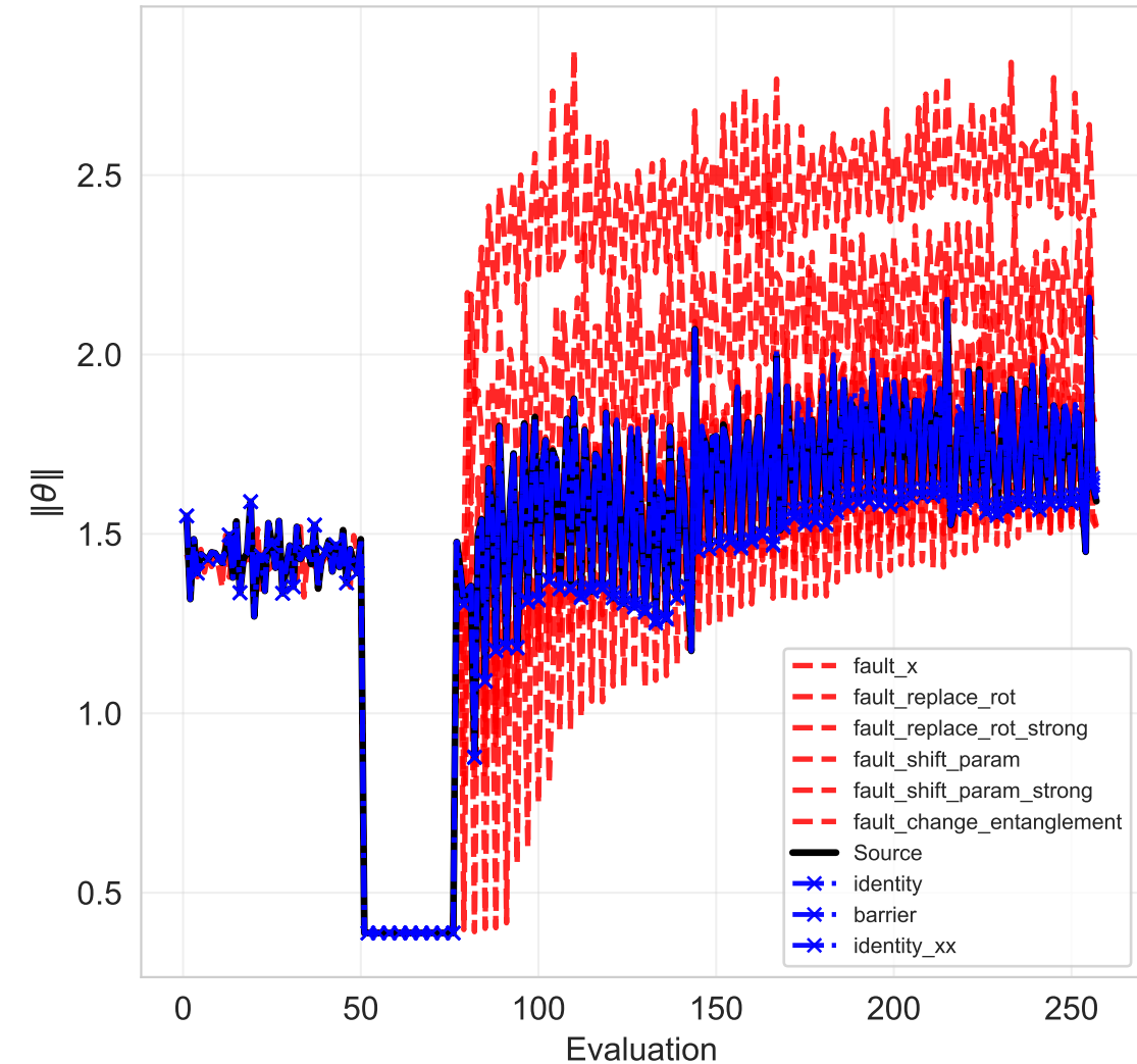
Noisy Parameter Norm Evolution
