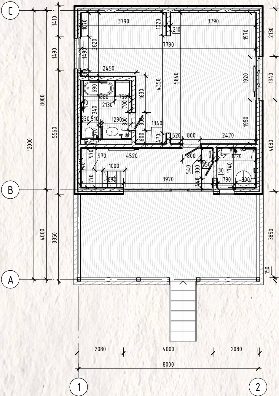
Кладочный план на отм. 0.000 (1:100)
