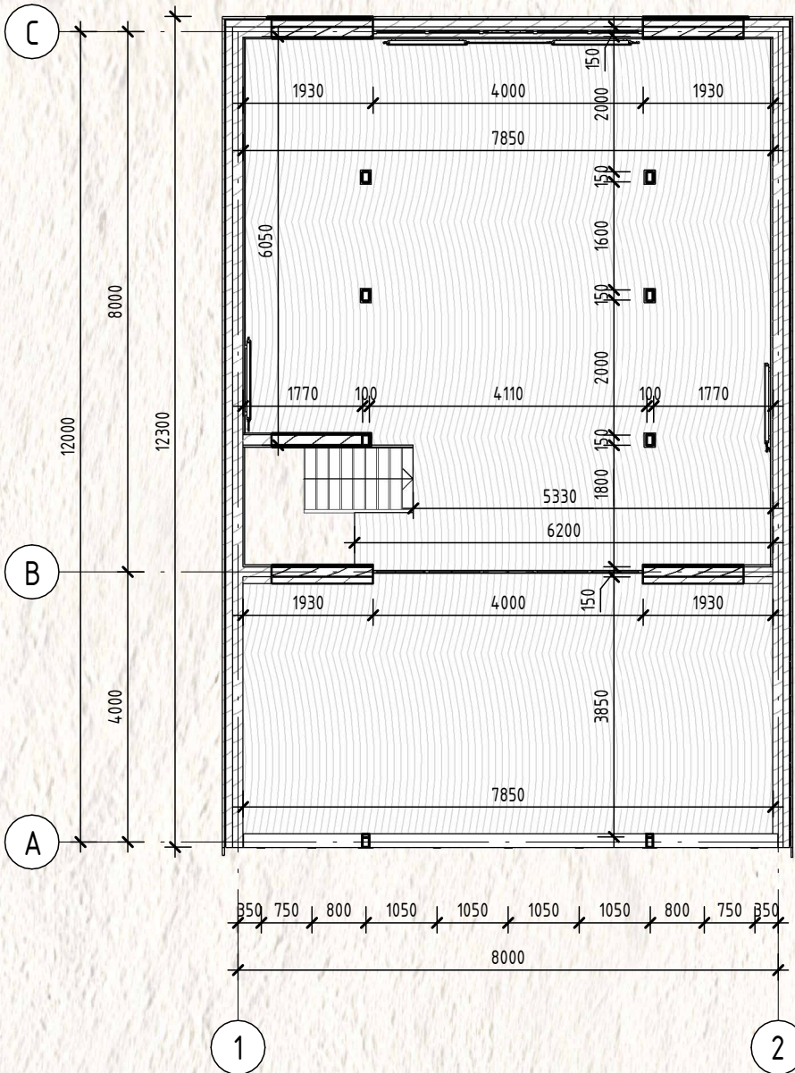
Кладочный план на отм. +3.000 М1:100
