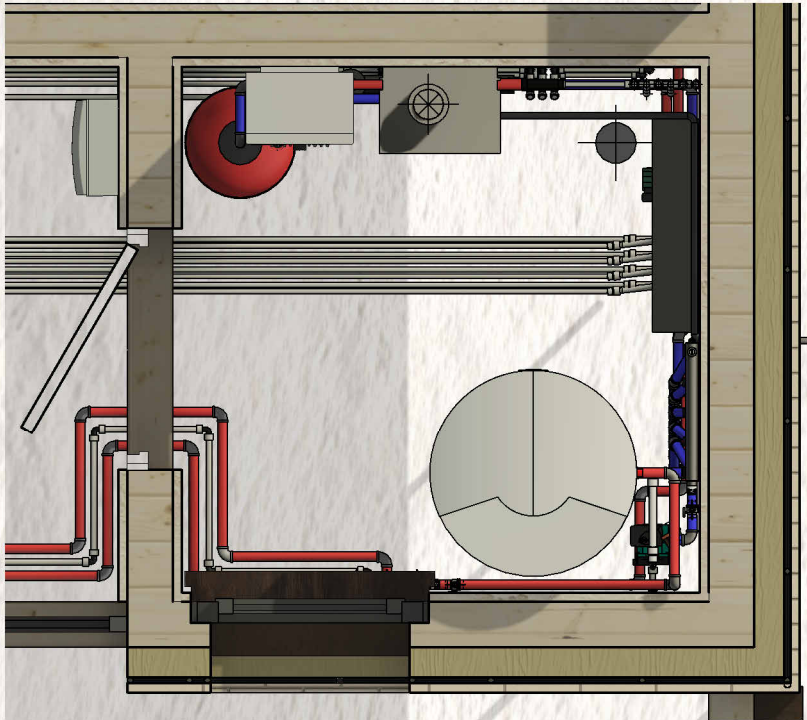
План расстановки оборудования помещения Котельной (1:25)
