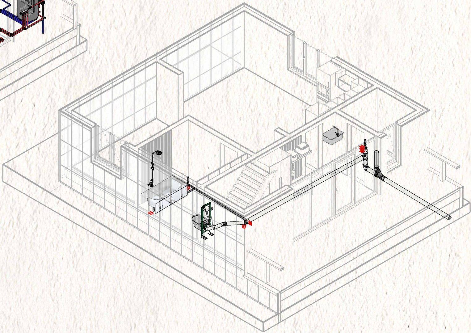
Схема системы канализации (К1)
