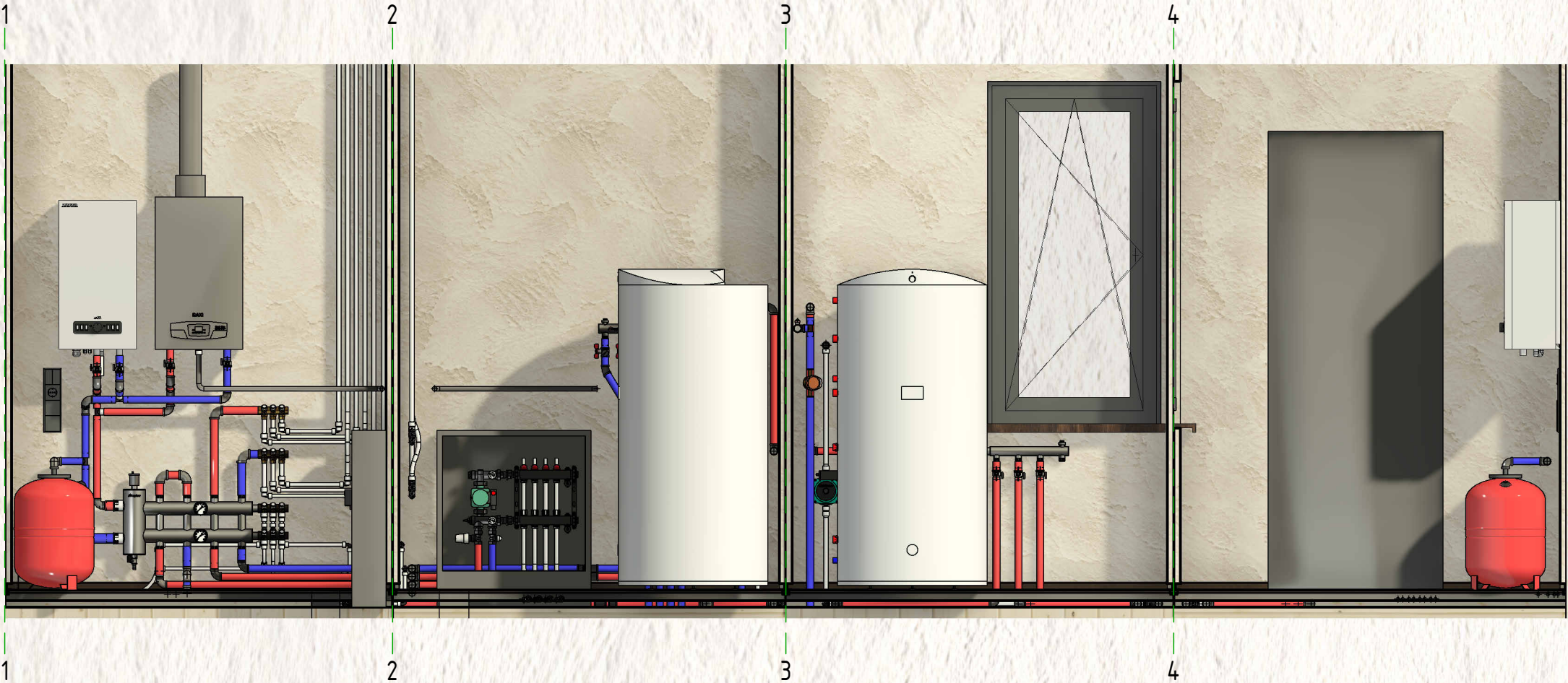
Развертка стен помещения Котельной (1:25)
