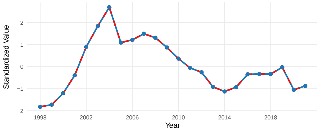
11.PredMammalSmolt_DFA1
