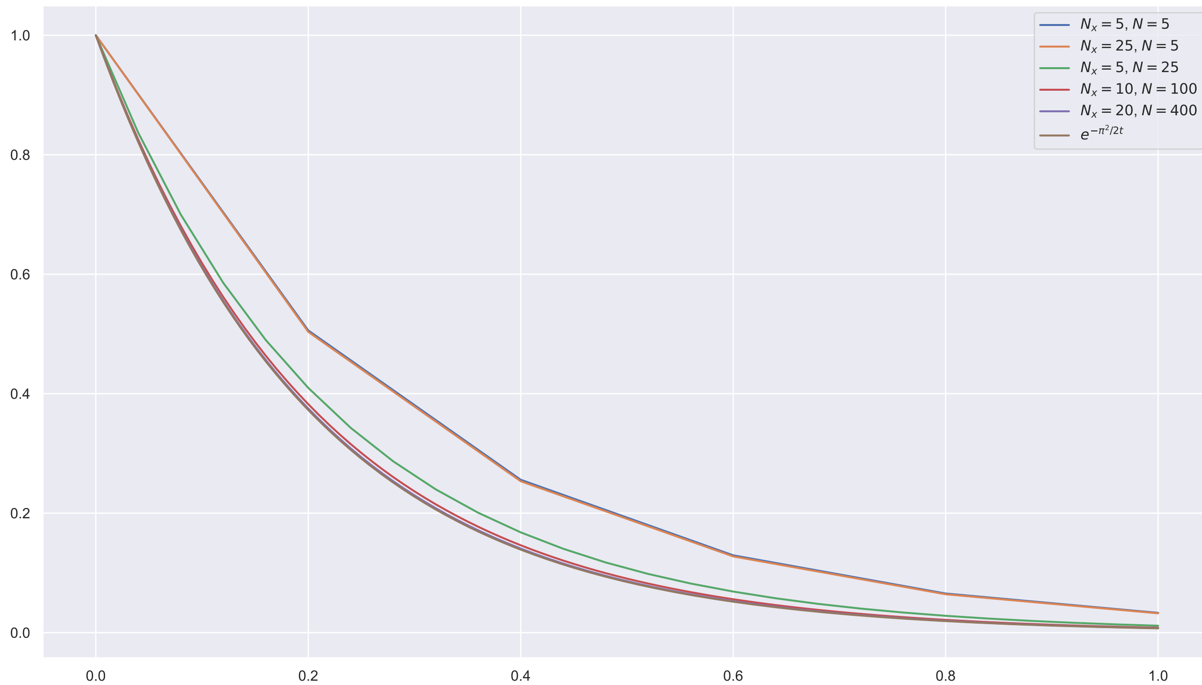
Коэффициент Фурье при базисной функции \sin(\pi/2x)\sin(\pi/2y)
