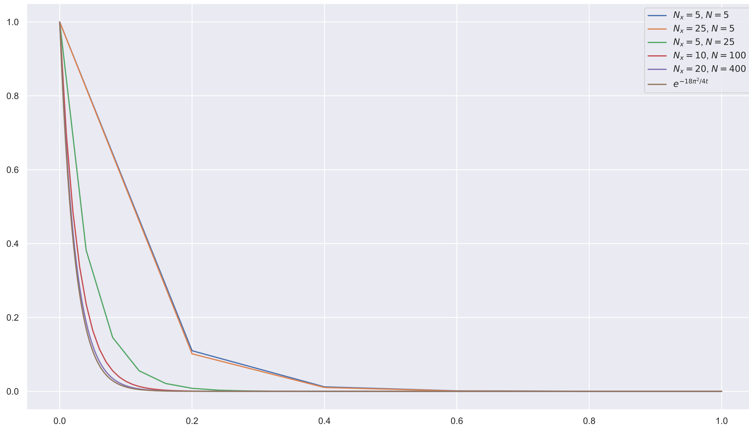
Коэффициент Фурье при базисной функции \sin(3\pi/2x)\sin(3\pi/2y)
