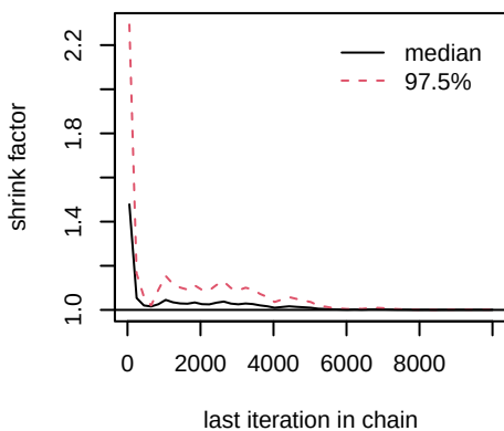
tau.1.
