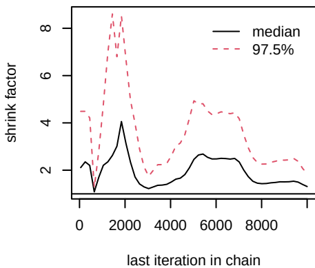
kapJ.1.
