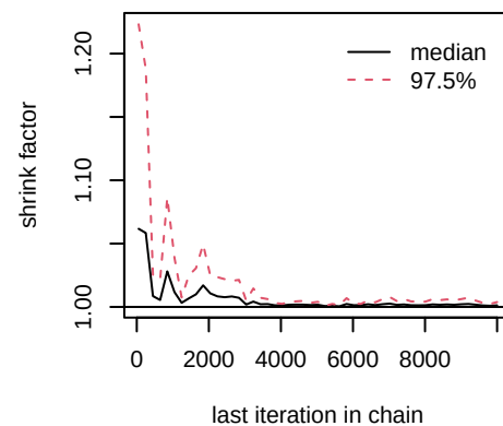
r_pAm_pM.1.
