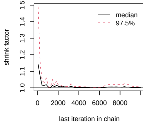
pAm.1.
