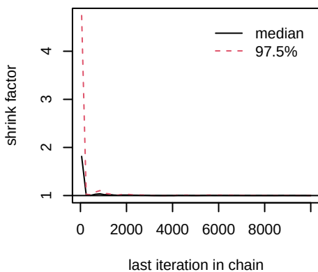
kJ.1.
